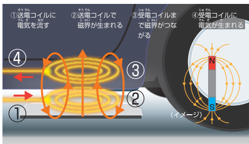
EV(電気自動車)向けワイヤレス充電システム
